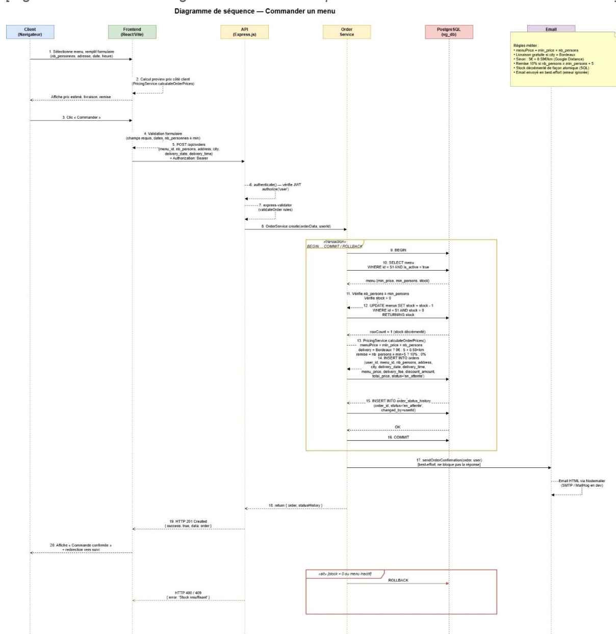
Figure 4 — Diagramme de séquence : commander un menu
