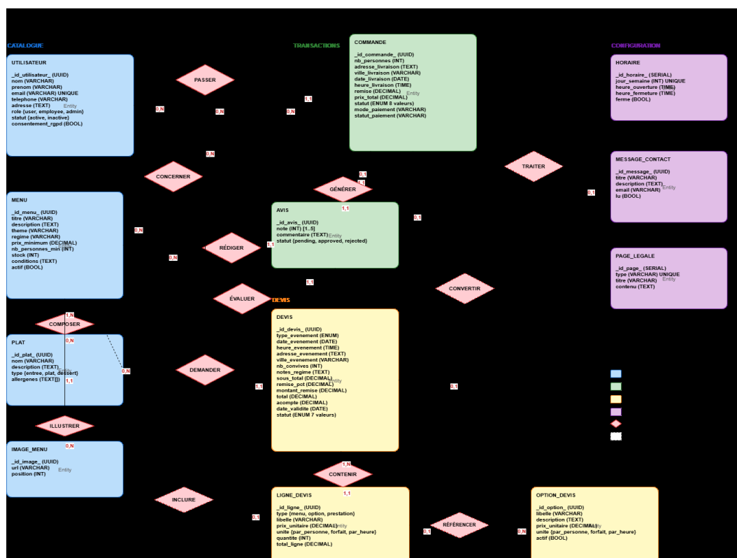
Figure 2 — Modèle Conceptuel de Données (MCD)
