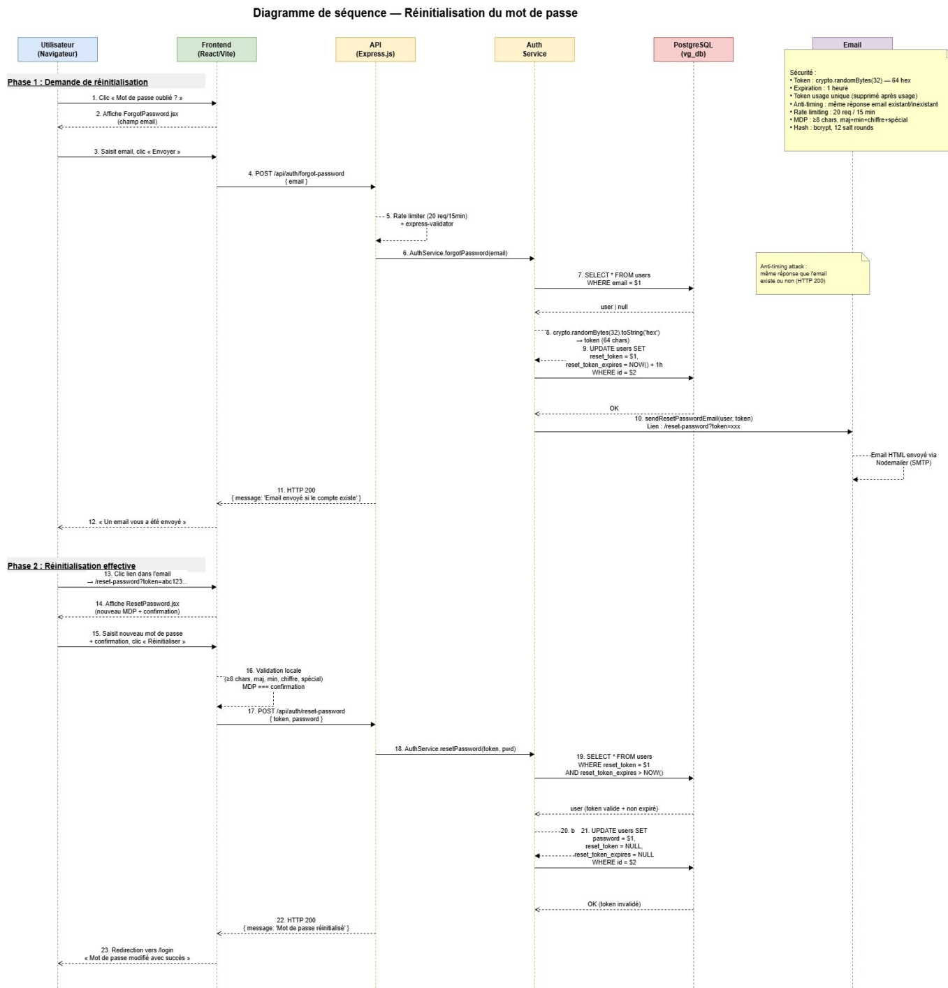
[Figure 5 — Diagramme de séquence : réinitialisation du mot de passe]
